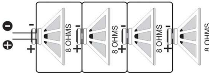
PARALELO 2 OHMS
